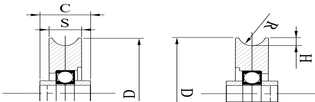
Poulie en Acier 1 Gorge R-10 1 Canal R-10 Steel Pulley
