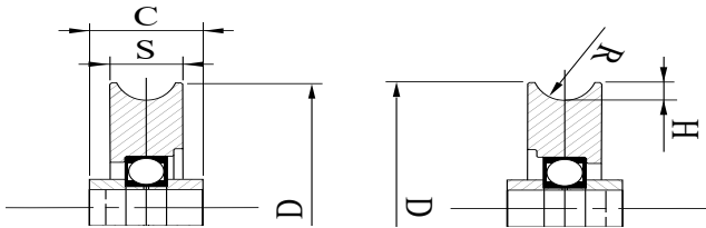
Poulie en Acier 1 Gorge R-10 1 Canal R-10 Steel Pulley
