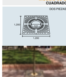
Modelo 03-B CUADRADO
